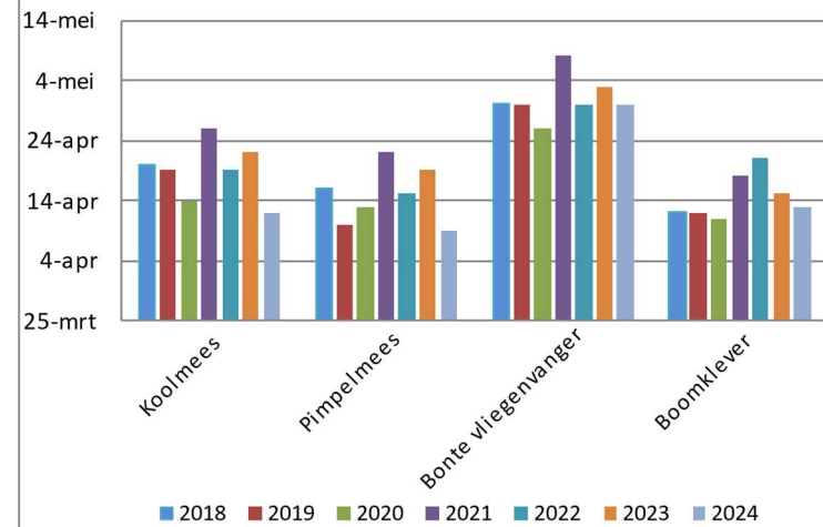
Trend Gemiddelde 1e ei datum zangvogelnestkasten Berkelland
