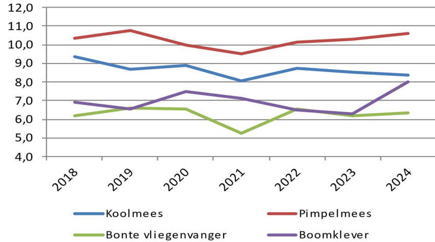
Trend Aantal eieren per legsel zangvogelnestkasten Berkelland
