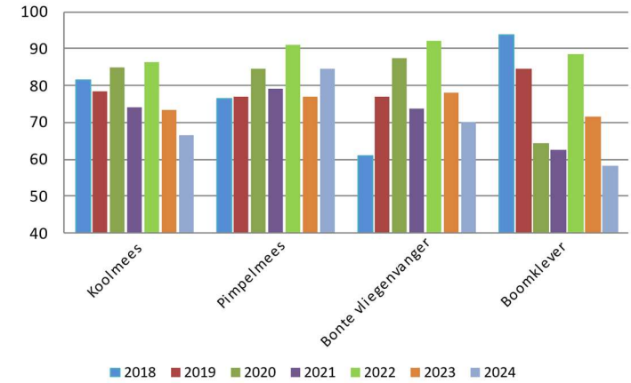
Trend % uitgevlogen jongen/eieren zangvogelnestkasten Berkelland
