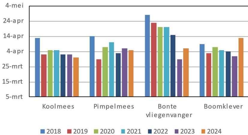
Trend 1e ei datum zangvogelnestkasten Berkelland
